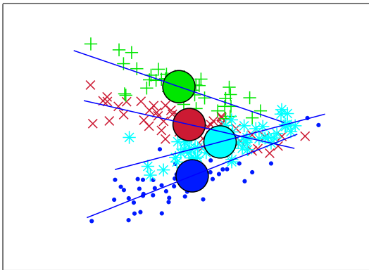
Fig. 14. Etape n°10 de l'HDDC sur les données « Crabes ».
